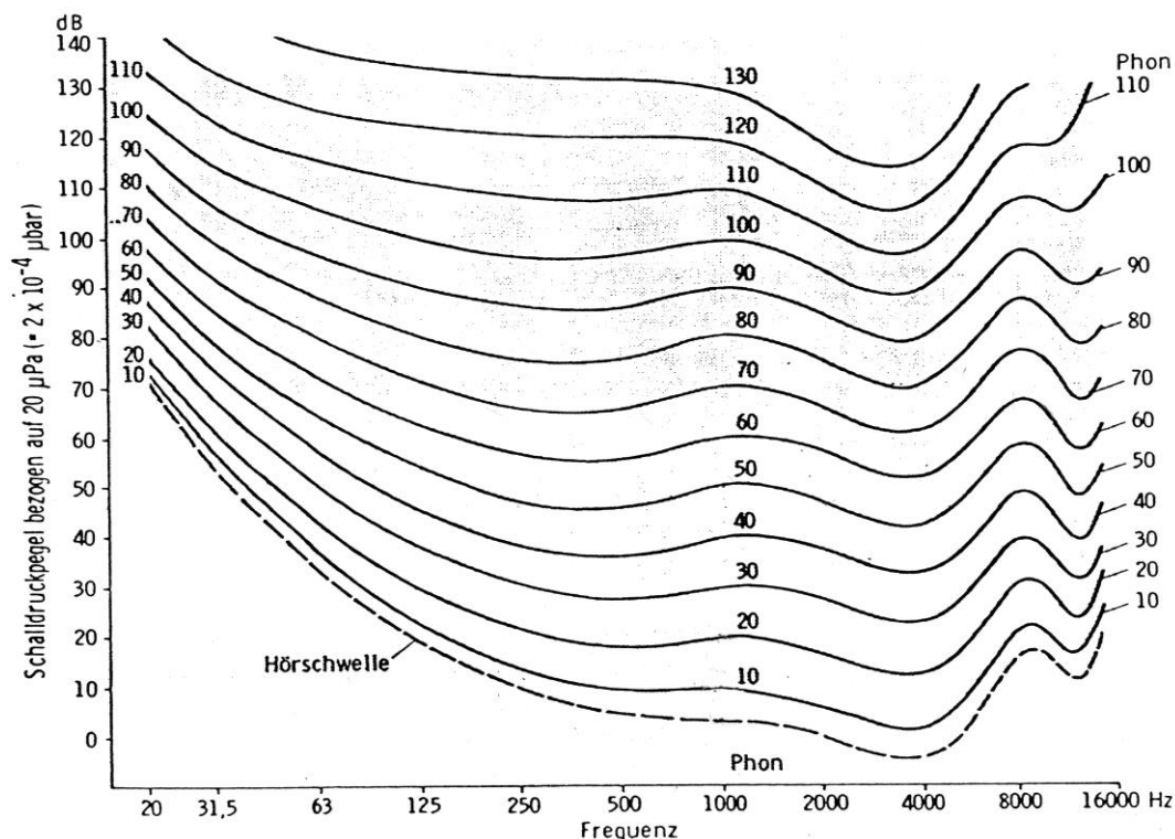
Abb 1: Historisches Isophonendiagramm nach Fletcher-Munson, ehemals DIN 45 630 ISO R 226.
